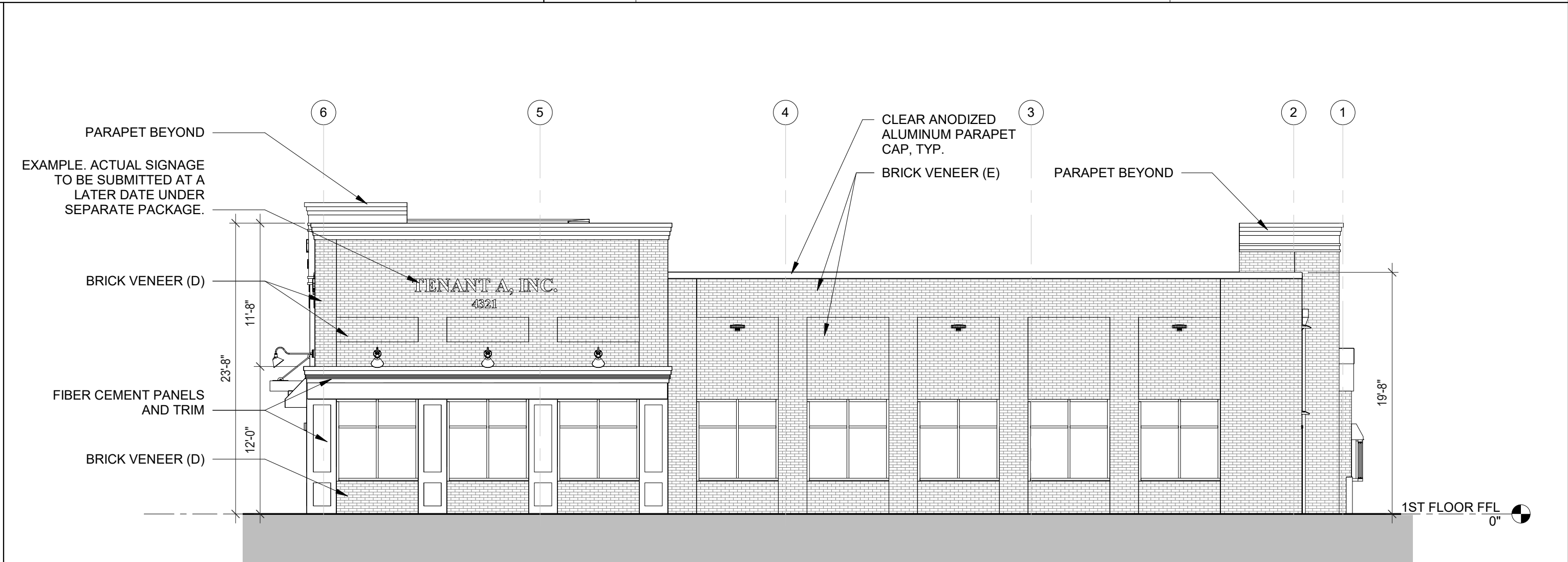
A5 EXTERIOR ELEVATION - NORTH CANOPY 1/8" = 1'-0"
