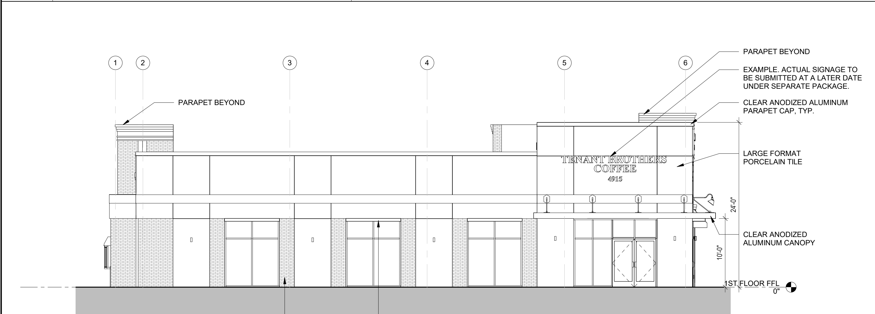
A1 EXTERIOR ELEVATION - EAST 1/8" = 1'-0"
