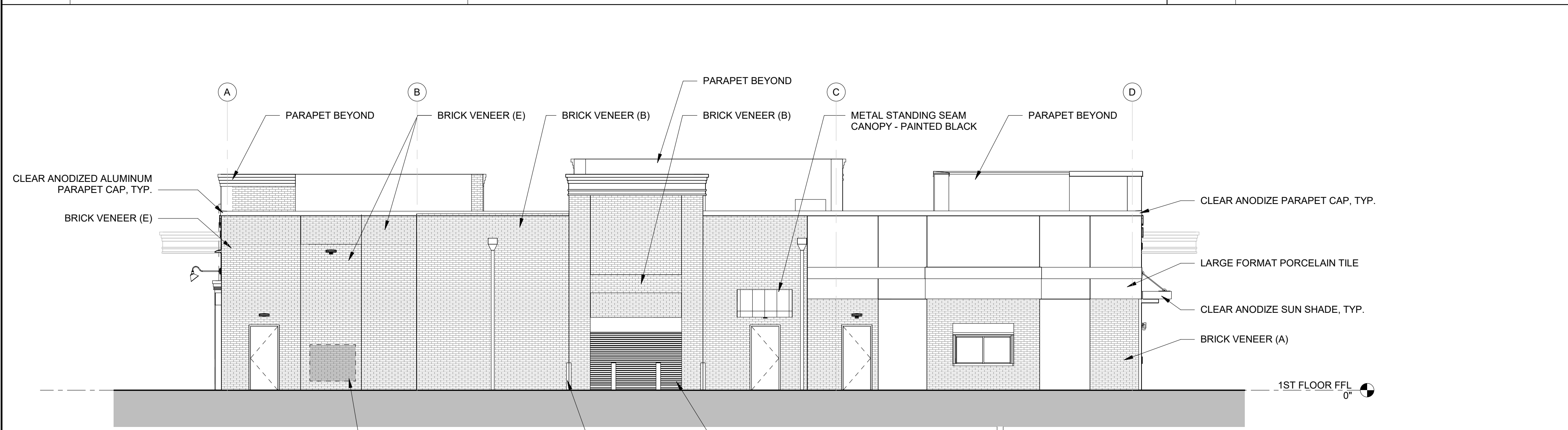
D1 EXTERIOR ELEVATION - WEST 1/8" = 1'-0"
